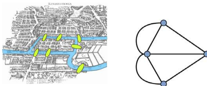
Mapa y puentes de Königsberg Fuente: BogdanGiușcă / CC-BY-SA-3.
